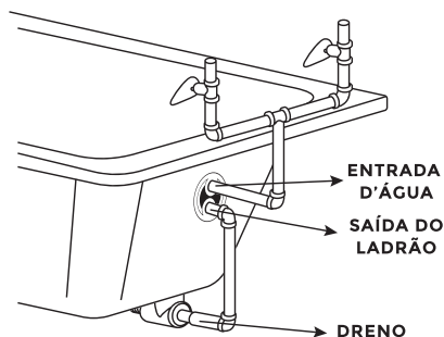
ILUSTRAÇÃO DE HIDRÁULICA COM MISTURADORES E SAÍDA DO DRENO
