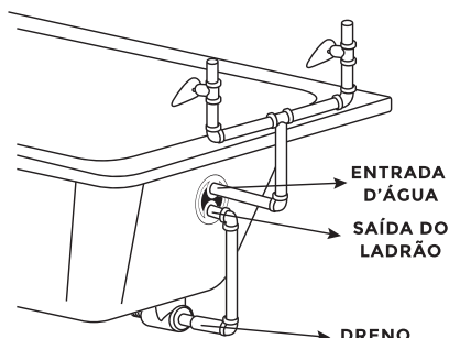
ILUSTRAÇÃO DE HIDRÁLICA COM MISTURADORES E SAÍDA DO DRENO
